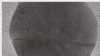
Au Nanoparticles
